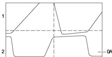
Dynamische Lastreaktion ohne Stromsenke: negativer Laststrom durch Rückinspeisung entsteht
